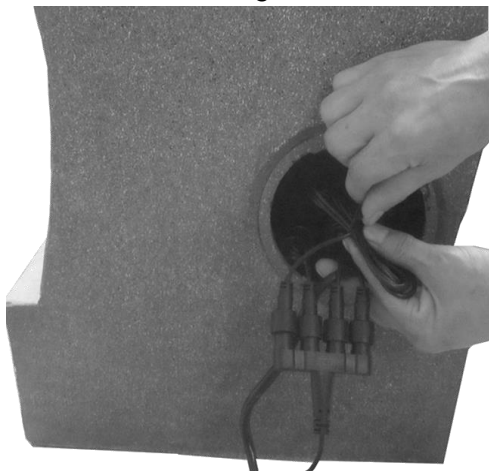
Trouver la connexion la lumière à l'intérieur de la fontaine. La connexion de la lumière doit rester en dehors de la fontaine.
